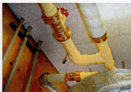
撮影項目 宿毛育成園給湯設備改修工事 ボイラー室給湯新規配管、支持、バルブ取付状況
