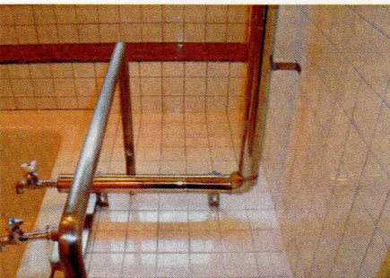
撮影項目 宿毛育成園給湯設備改修工事 浴室南側バス水栓ステン配管ラッキング状況
