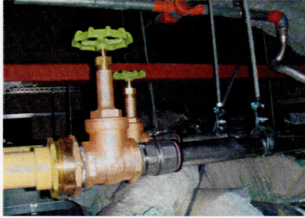
撮影項目 宿毛育成園給湯設備改修工事 西側 南廊下天井内給湯配管、バルブ取付配管、支持状況
