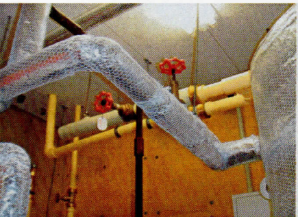
撮影項目 宿毛育成園給湯設備改修工事 ボイラー室給湯新規配管、支持、バルブ取付状況
