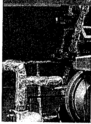
撮影項目 宿毛青成園ボイラー室 給湯配管改修工事 ボイラー室新設改修配管 保温被覆
